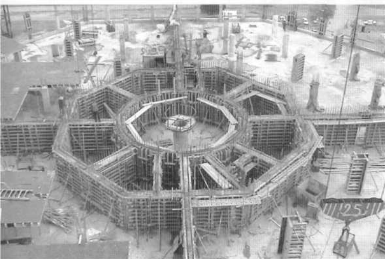
Рисунок 11. Опалубка ядра и диафрагм жесткости типового этажа
