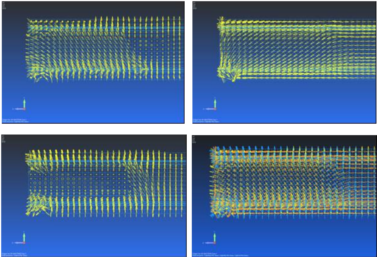
Рисунок 6. Траектории главных напряжений
