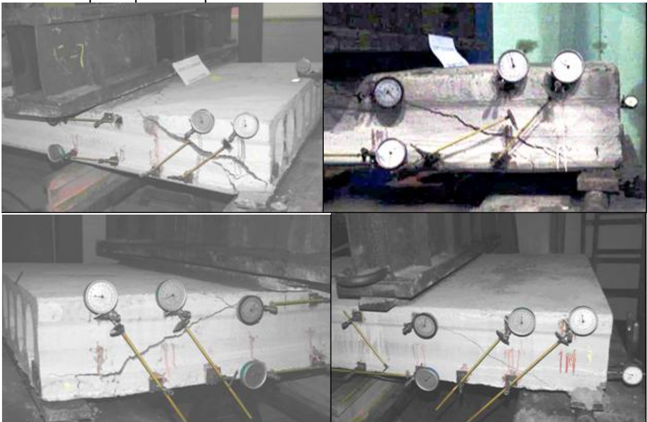
Рисунок 9 – Общий вид разрушения плит 1-й серии по наклонным сечениям при испытаниях на сдвиг
