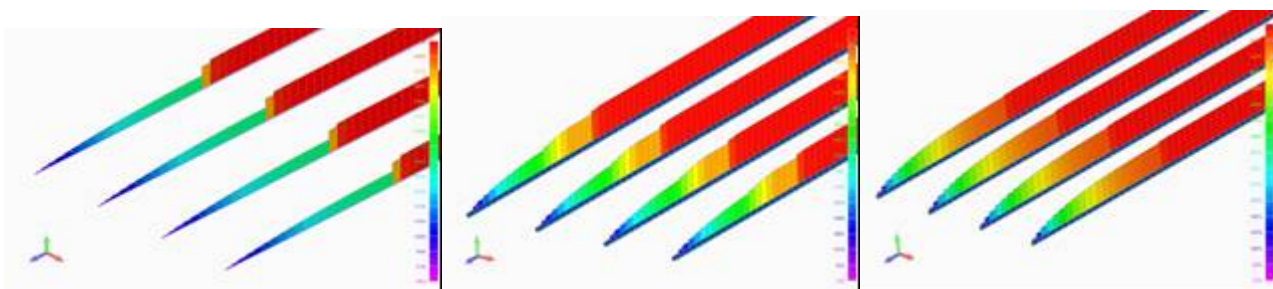
Рисунок 4. Распределение напряжений по длине зоны передачи напряжения канатов при различных законах «усилие – перемещение»
