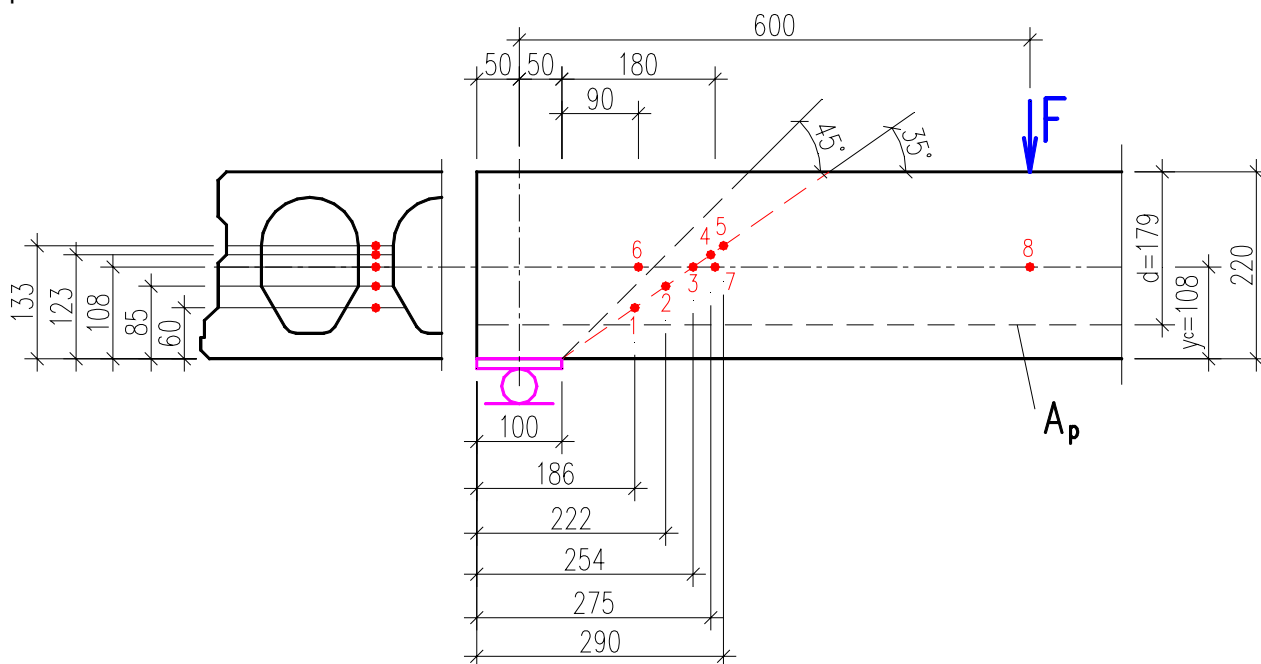
Рисунок 7 - Расчетная схема плиты по определению прочности наклонного сечения на сдвиг
