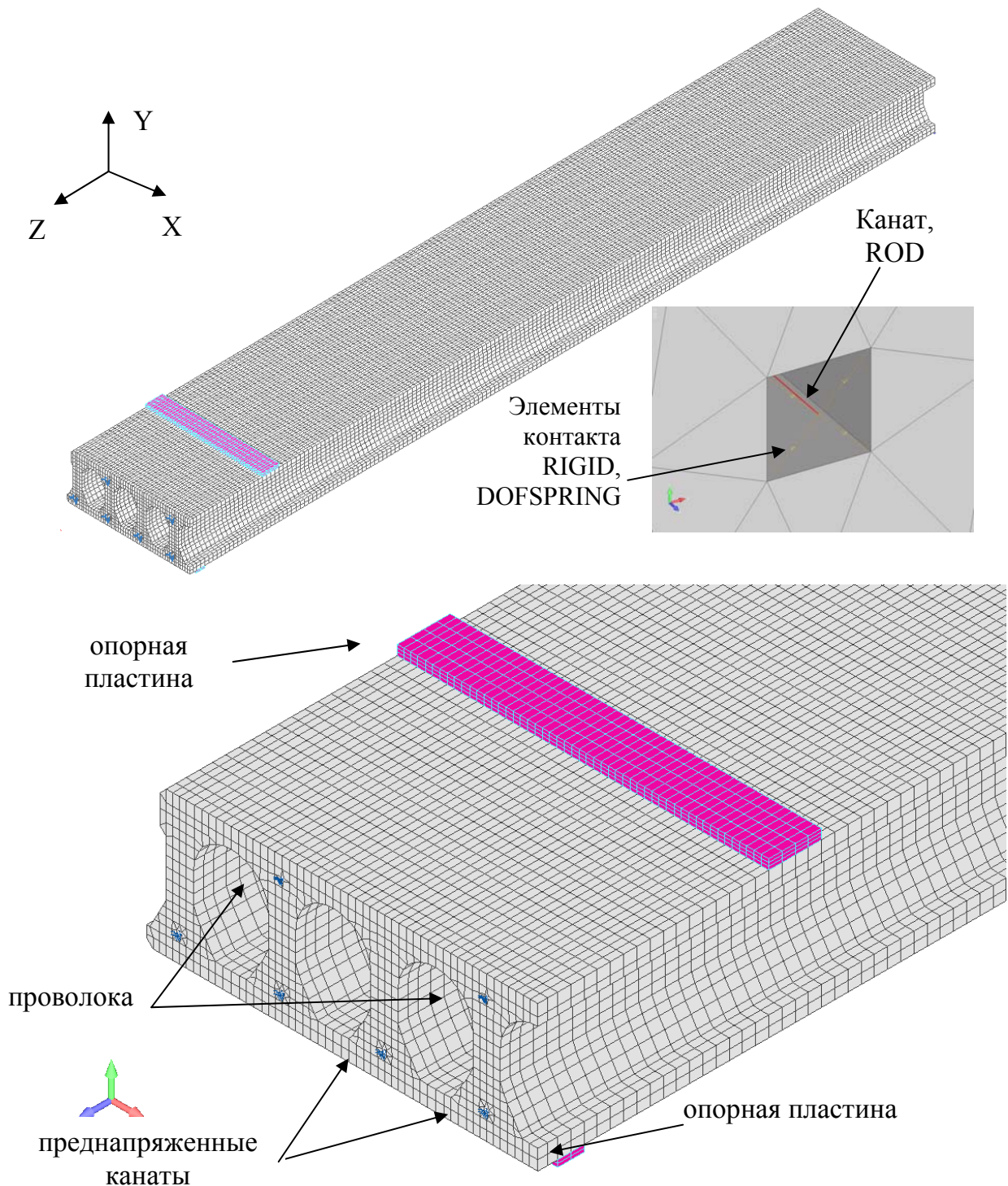
Рисунок 1 - Общий вид расчетной модели и ее фрагмента
