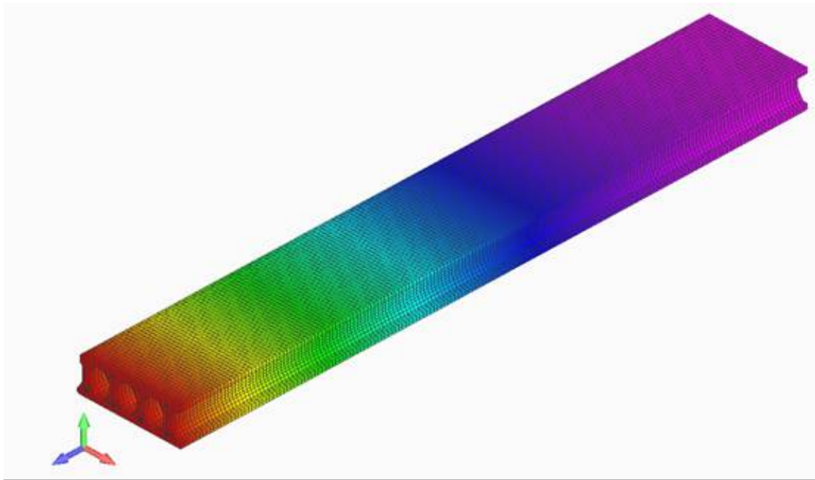
Рисунок 2. Деформированная схема плиты
